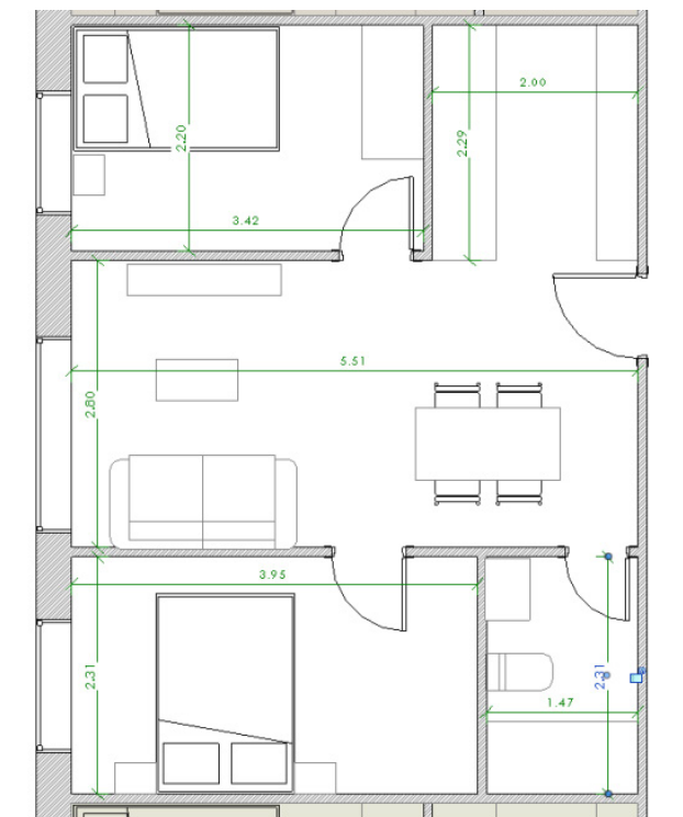
Plano apartamento 2 habitaciones.
