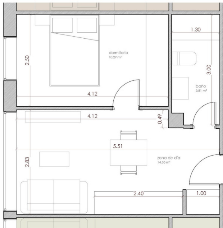
Plano apartamento 1 habitación.
