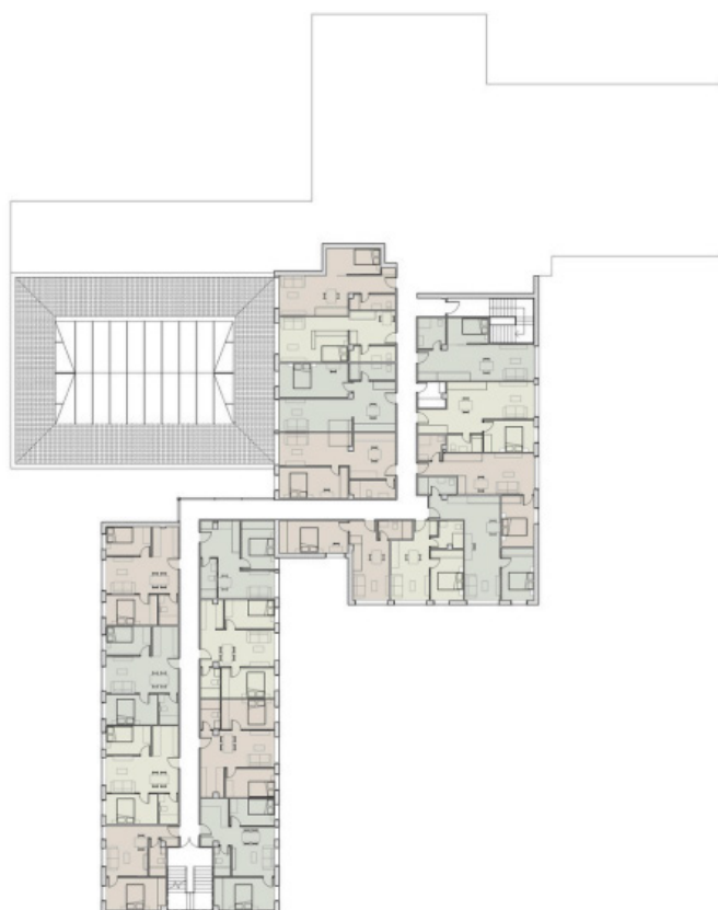
planta segunda
